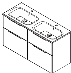
Dupla kerámiamosdó, 100x46,5 cm
